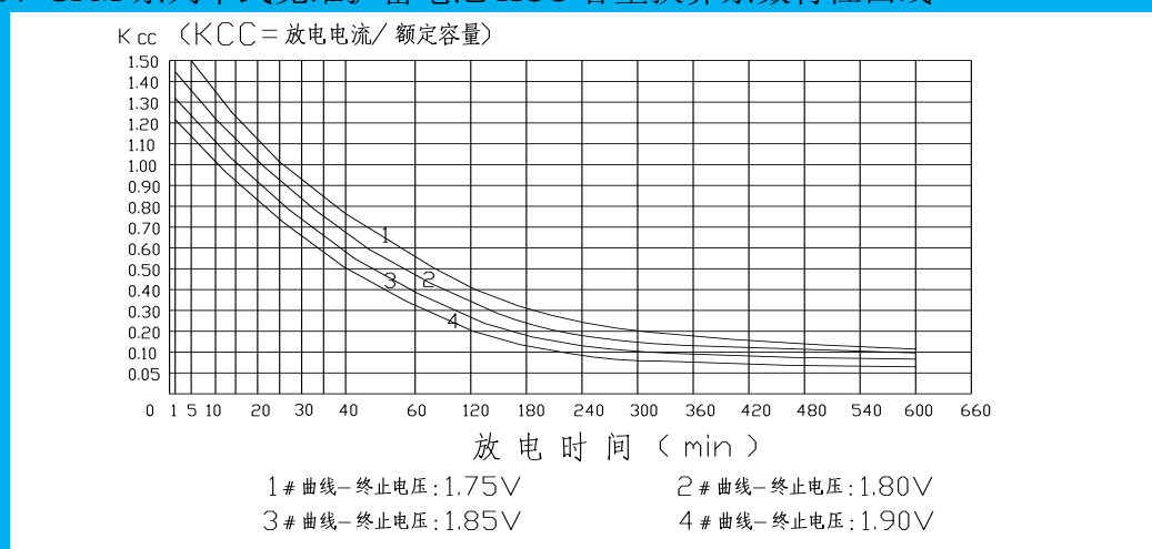
8、GFM 系列干式免维护蓄电池 KCC 容量换算系数特性曲线
